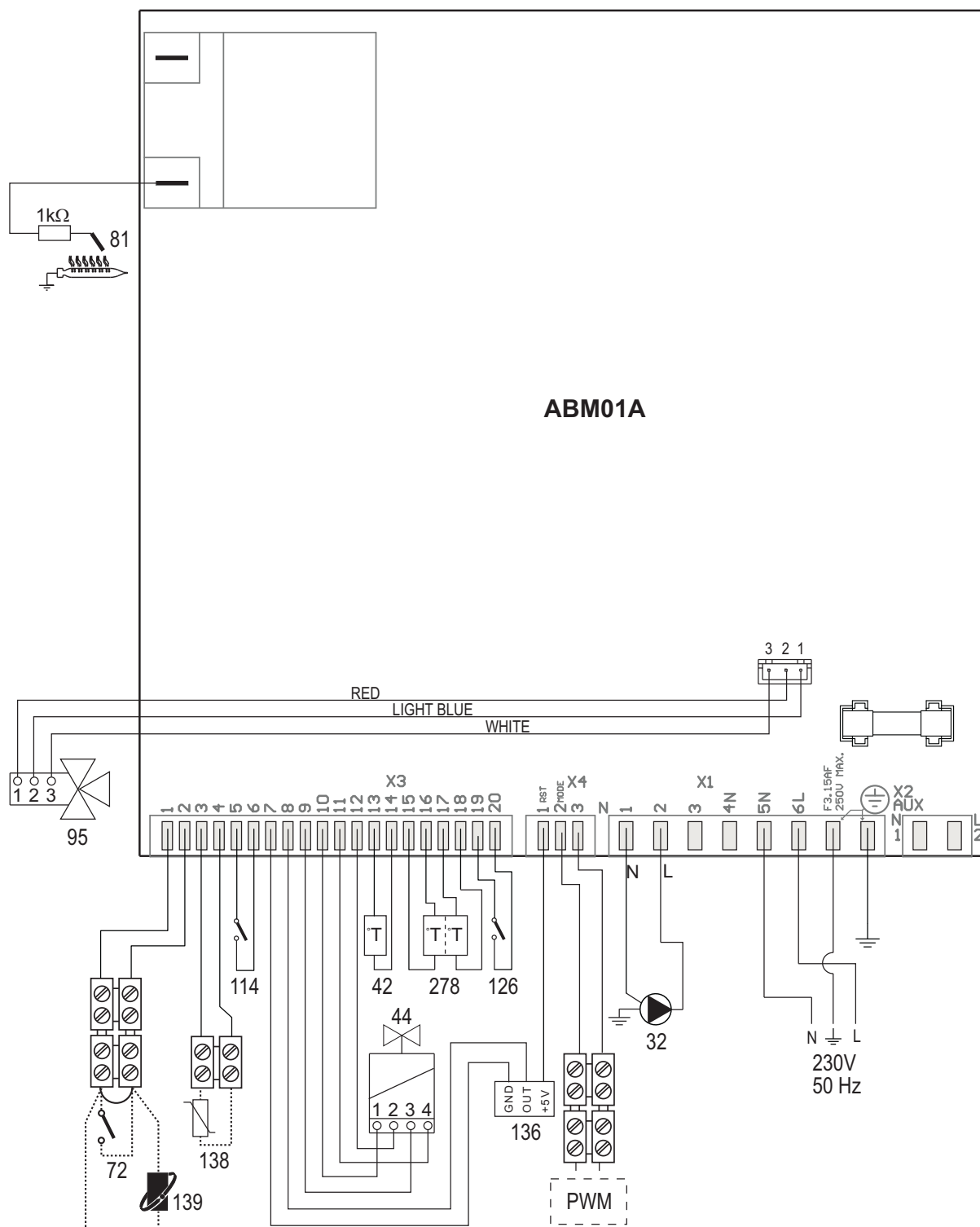
fig. 23- Schéma électrique
