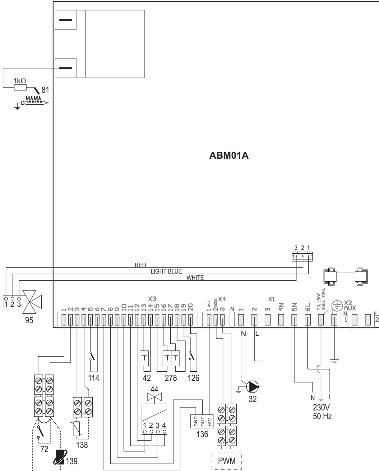
fig. 23 - Schema elettrico
