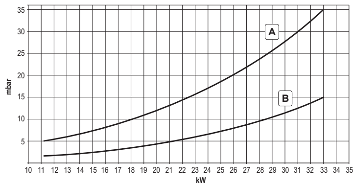
Diagrammes pression - puissance DIVAtch D LN C30
