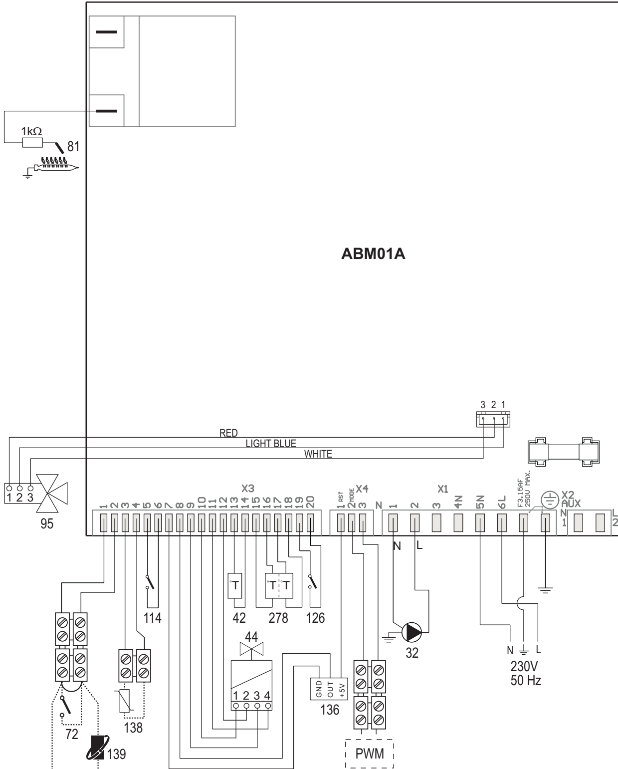
fig. 23- Wiring diagram
